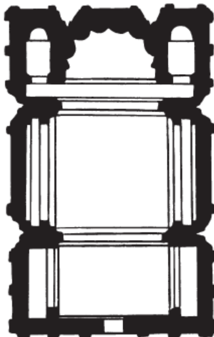
Рис. 24. Ахтамар. Церковь Святого Креста. 915-921 гг. (по Хачатряну), 1:350
