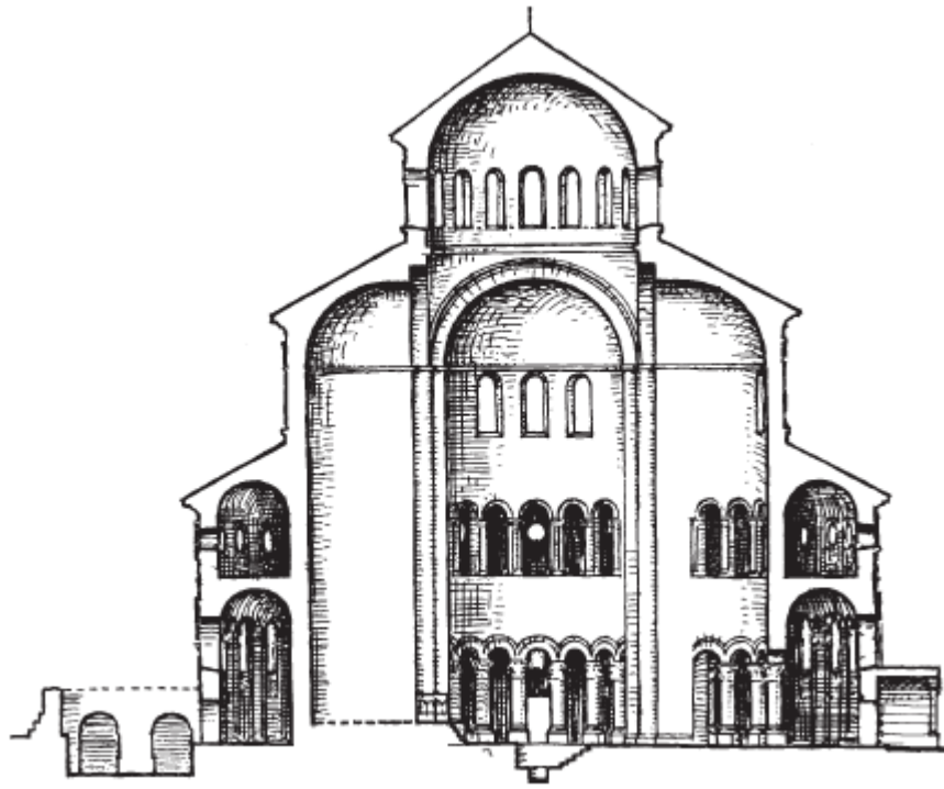
Рис. 18. Секционный вид церкви Звартноц (рисунок Кеннета Дж. Конанта)
