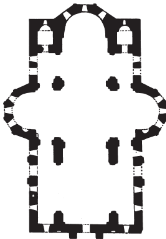
Рис. 14. Собор в Мрене. 638-640 гг. 1:500
