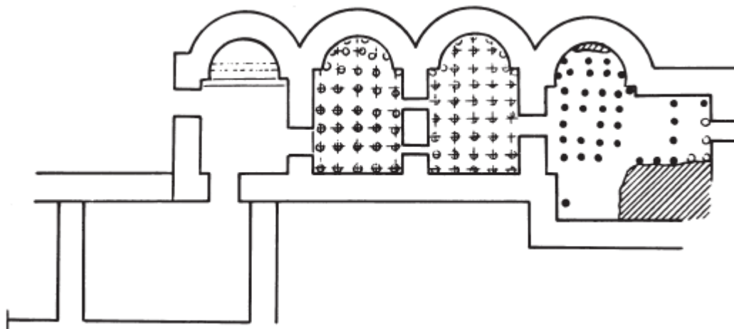
Рис. 10. План бань Гарни (по Аракеляну)
