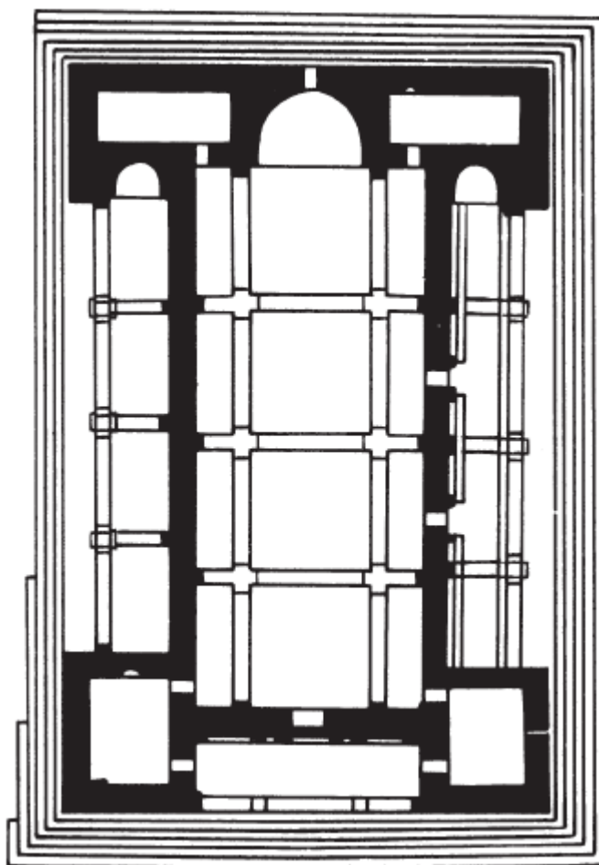
Рис. 12. Базилика Ереука. V-VI вв. (по Хачатряну)
