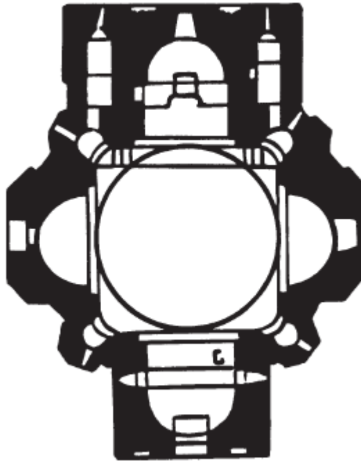
Рис. 24. Ахтамар. Церковь Святого Креста. 915-921 гг. (по Хачатряну), 1:350
