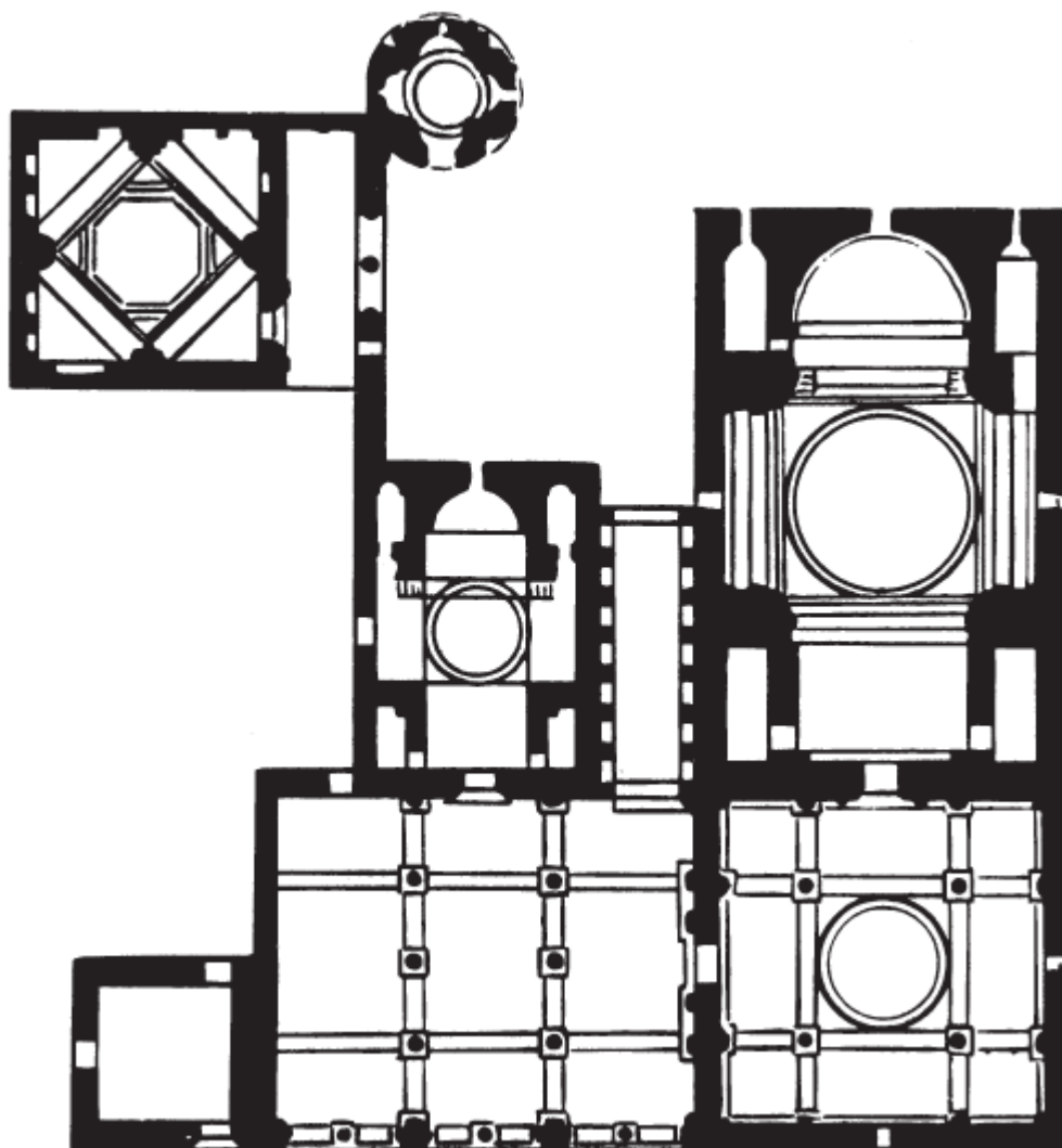
Рис. 26. Монастырь в Санахине: 1 - церковь Божьей Матери. X в.; 2 - церковь Спасителя. 966 г.; 3 - сводчатый зал, известный как Академия Григория Магистра; 4 - часовня Святого Григория. 1061 г.; 5 - библиотека. 1063 г.; 6 - гавит (жаматун). 1181 г.; 7 - гавит. 1211 г.; 8 - звонница.
