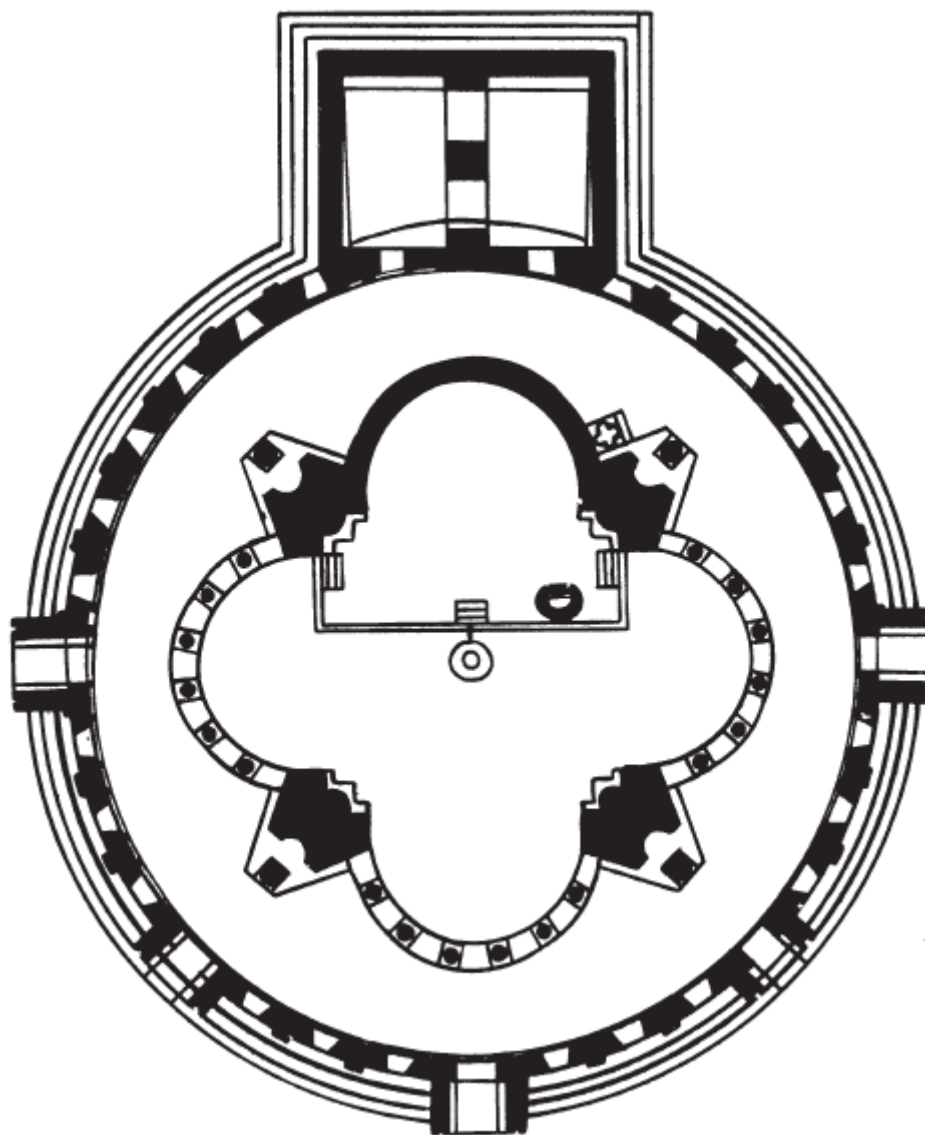
Рис. 17. План церкви Звартноц. 644-652 гг. (по Хачатрян), 1:500
