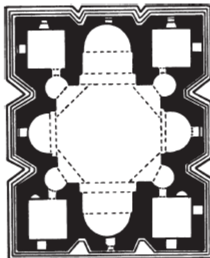
- Рис. 19. Вагаршапат. План церкви Святой Рипсимэ. 618 г. (по Хачатрян), 1:500
