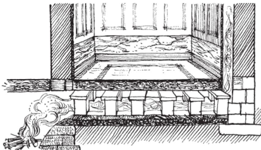
Рис. 2. Гипокауст - отопительная система в домах Древнего Рима
