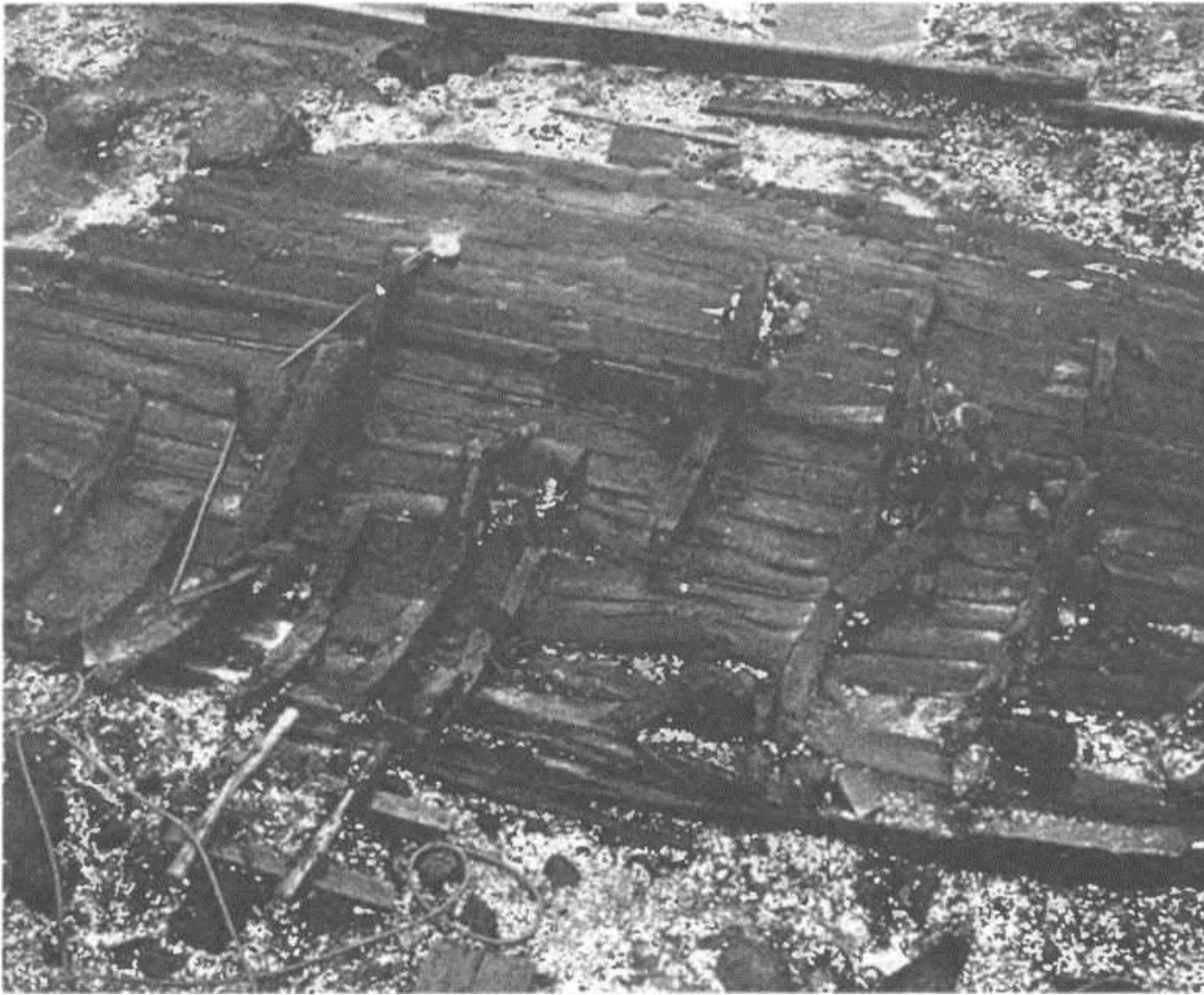
Корпус купеческого корабля, обнаруженного в Роскильде-фьорде [ *** ]
